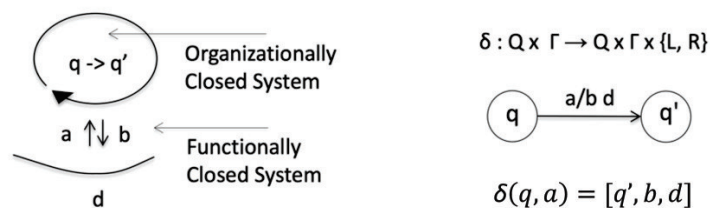
Figura 1: Equivalência da função de transição da máquina de Turing com o fechamento organizacional e funcional da máquina de Maturana & Varela.
