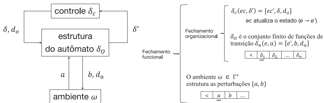
Figura 2: Arquitetura de uma máquina de Turing Enativa (MTE). Uma configuração da unidade discreta origina outra, [e, xacy] \vdash [e', xbcy] onde \delta(e, a) = [e', b, Direita] , em um processo que permanece a deriva. O ambiente é indissociável da configuração da MTE.
